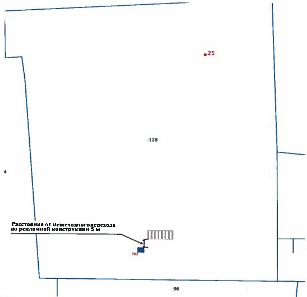
Топоъемка М 1:500
