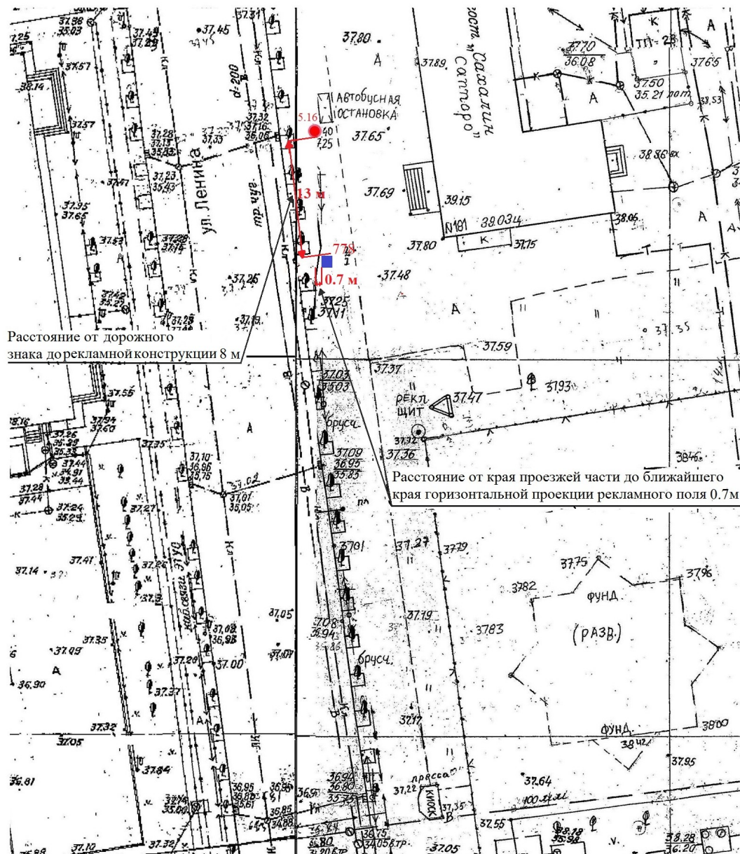
Топосъемка М 1:500
