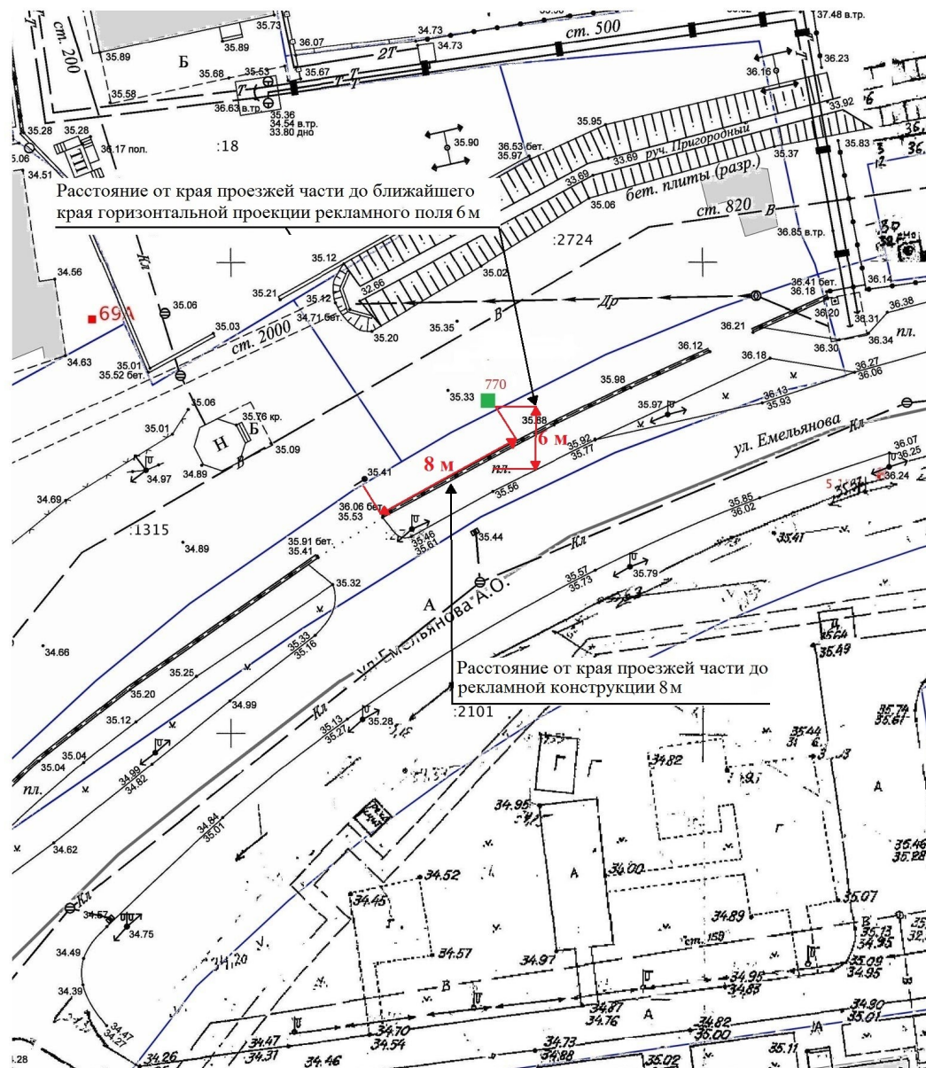
Топосъемка М 1:500
