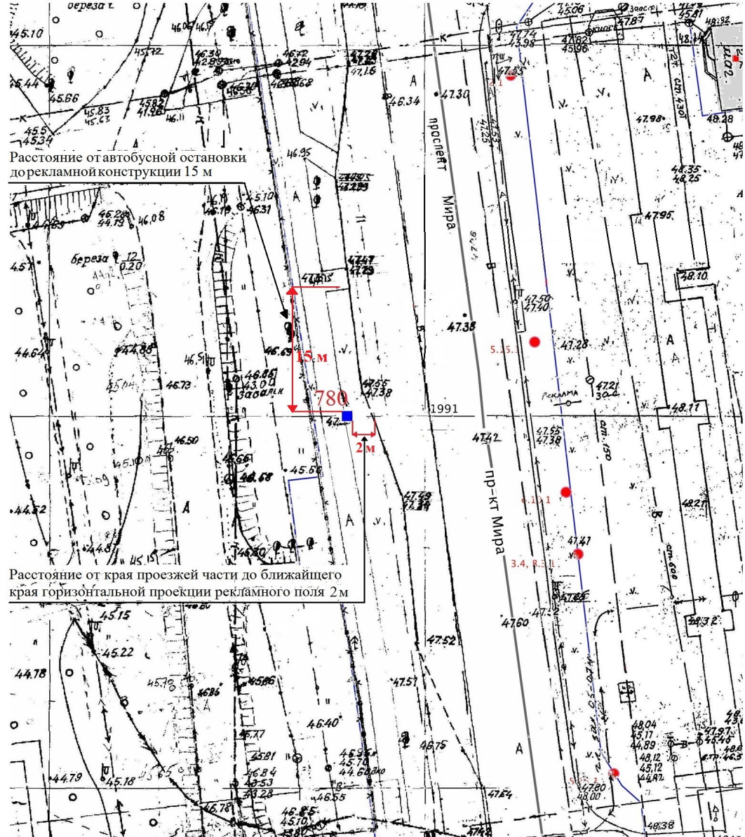
Топосъемка М 1:500
