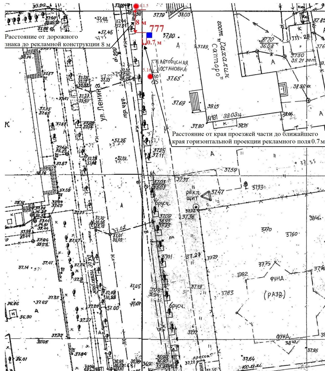
Топосъемка М 1:500
