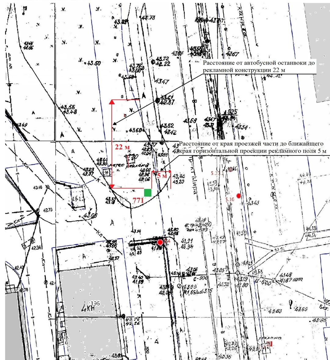
Топосъемка М 1:500
