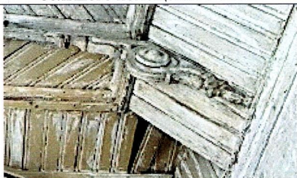
Резной кронштейн в интерьере восточного помещения 1 этажа
