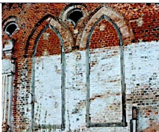
Ложные окна 1 этажа бокового фасада, выходящего в проулок
