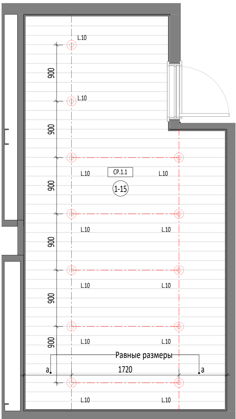
ПЛАН ПОТОЛКОВ С ПРИНЦИПИАЛЬНОЙ РАСКЛАДКОЙ МАТЕРИАЛА И РАССТАНОВКОЙ СВЕТИЛЬНИКОВ
