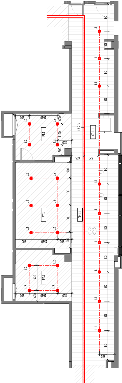
ПЛАН ПОТОЛКОВ С ПРИНЦИПИАЛЬНОЙ РАСКЛАДКОЙ МАТЕРИАЛА И РАССТАНОВКОЙ СВЕТИЛЬНИКОВ
