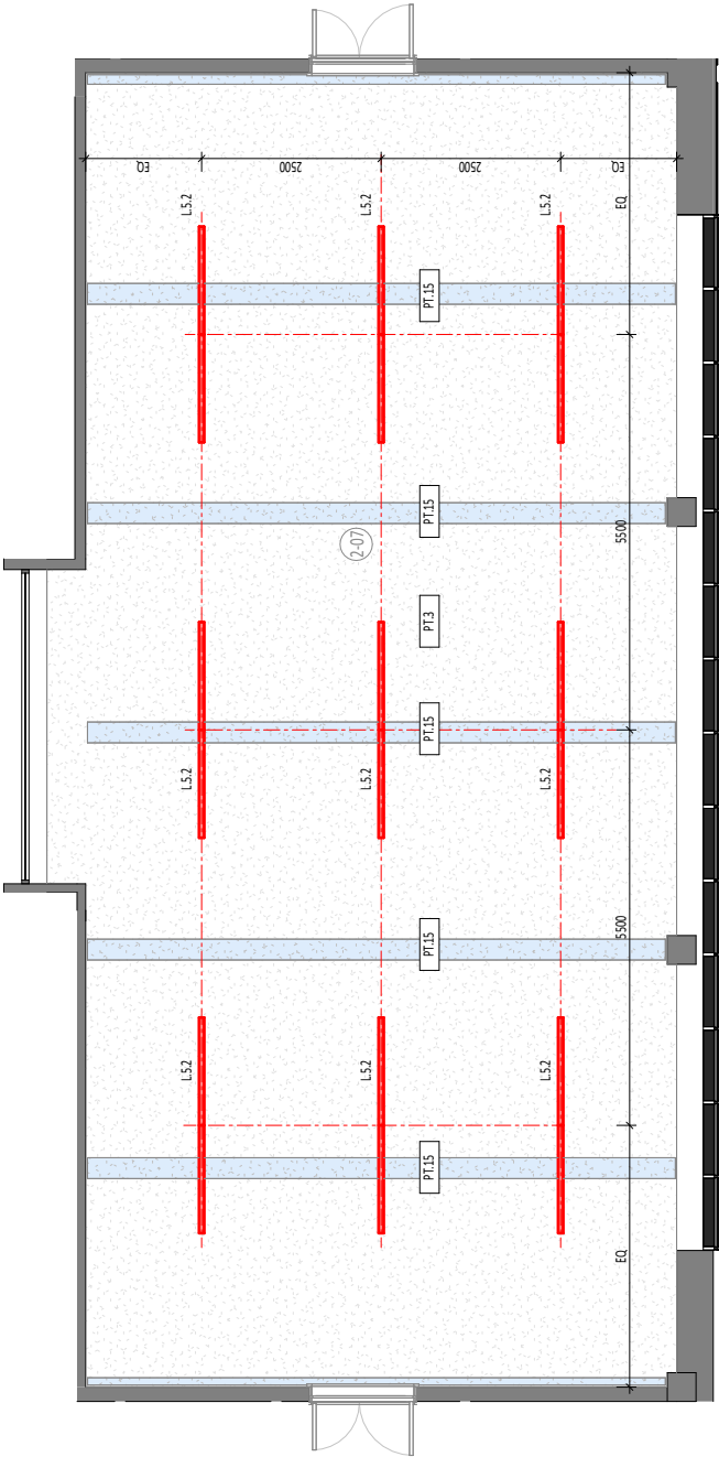
ПЛАН ПОТОЛКОВ С ПРИНЦИПИАЛЬНОЙ РАСКЛАДКОЙ МАТЕРИАЛА И РАССТАНОВКОЙ СВЕТИЛЬНИКОВ
