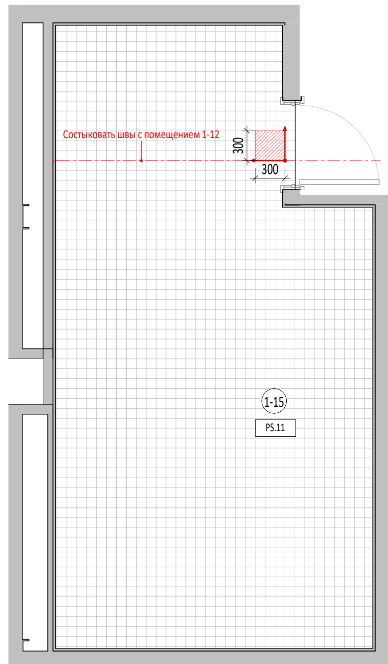
ПЛАН ПОЛОВ С ПРИНЦИПИАЛЬНОЙ РАСКЛАДКОЙ МАТЕРИАЛА
