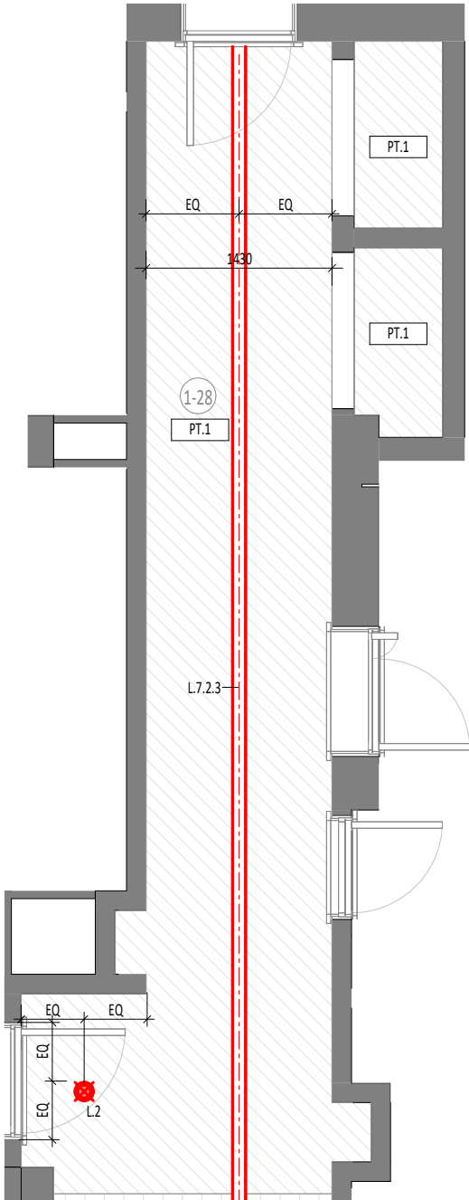
ПЛАН ПОТОЛКОВ С ПРИНЦИПИАЛЬНОЙ РАСКЛАДКОЙ МАТЕРИАЛА И РАССТАНОВКОЙ СВЕТИЛЬНИКОВ
