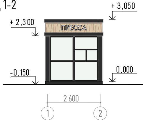
Схема плана
