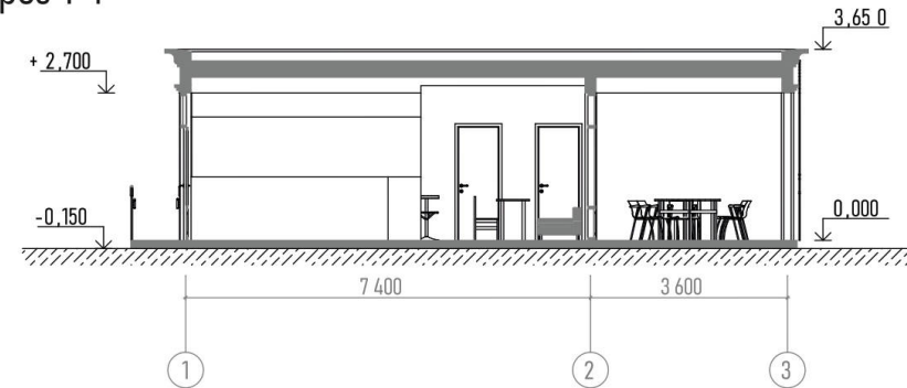
Разрез 1-1
