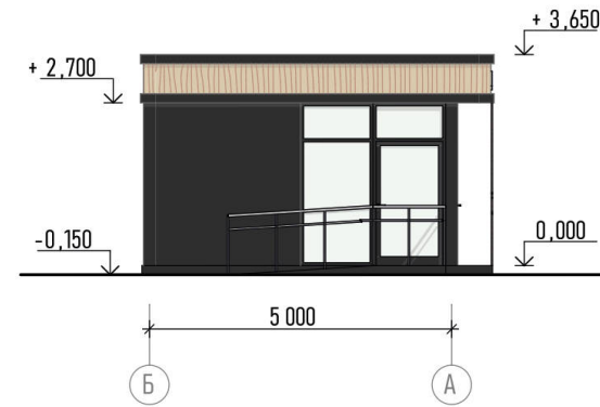
Фасад Б-А
