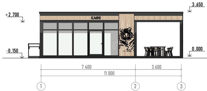
Фасад 1-3
