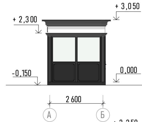
Фасад А-Б
