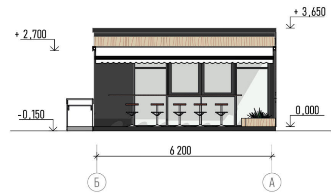
Фасад Б-А
