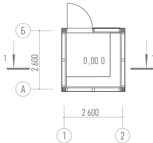
Схема плана
