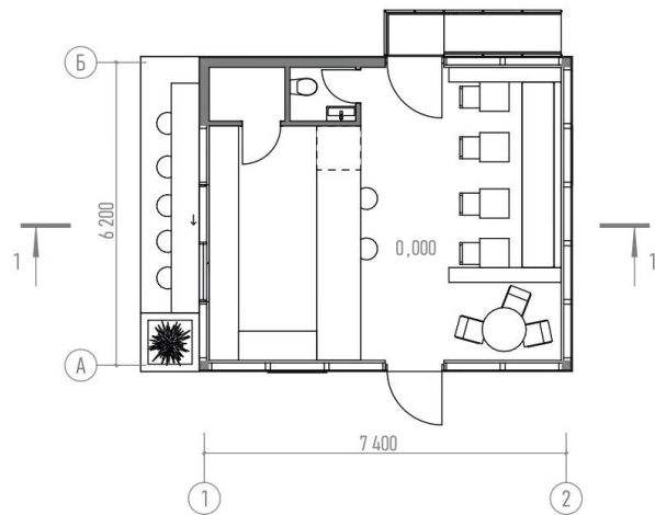
Схема плана
