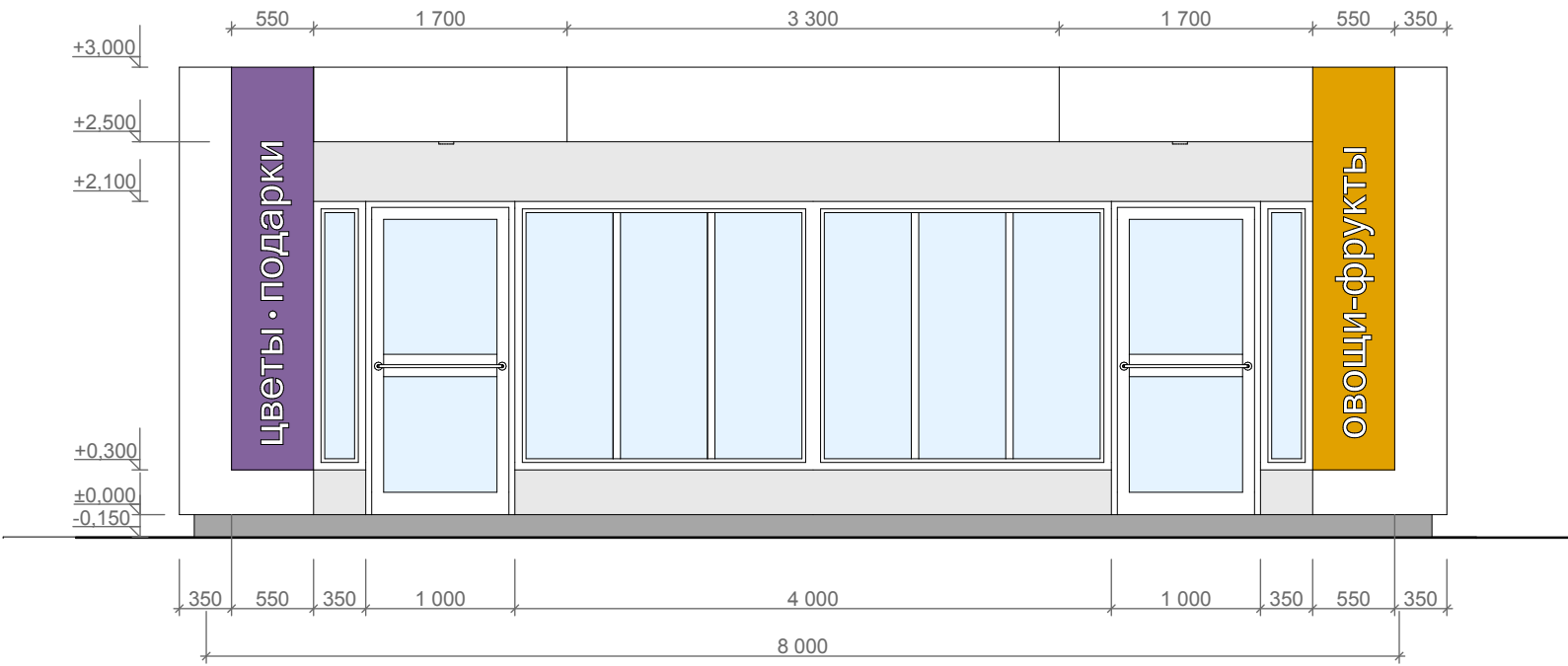
Главный фасад
