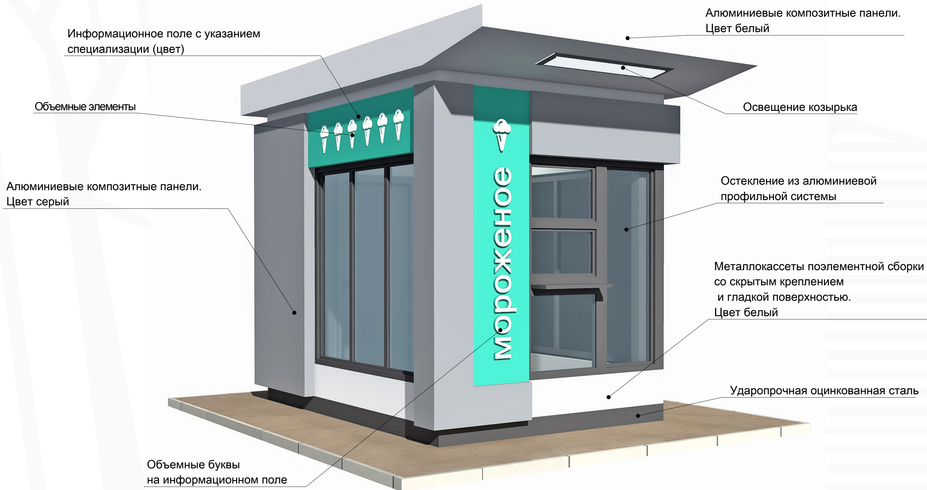
Внешний вид. Вариант с облицовкой композитными панелями для киоска «Мороженое». Размер в плане 2 x 3 м
