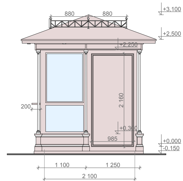
Боковой фасад
