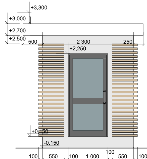
Боковой фасад
