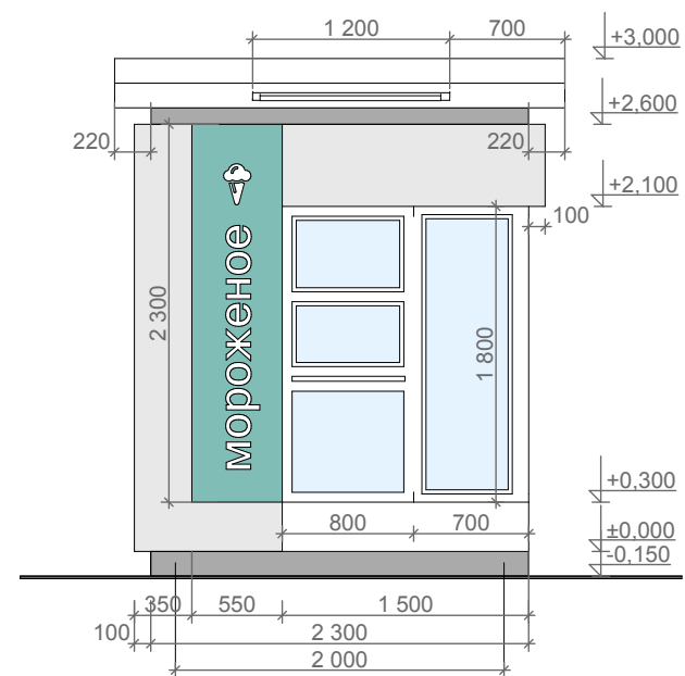
Главный фасад
