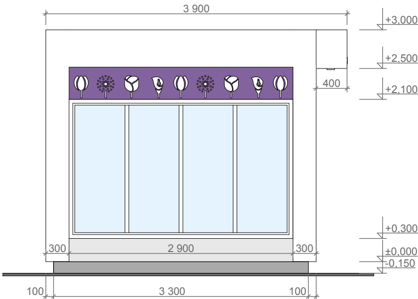
Боковой фасад
