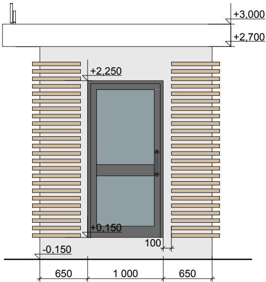
Боковой фасад
