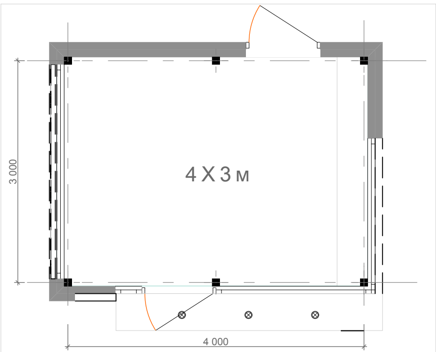
План
