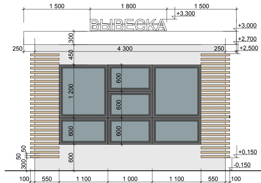
Главный фасад
