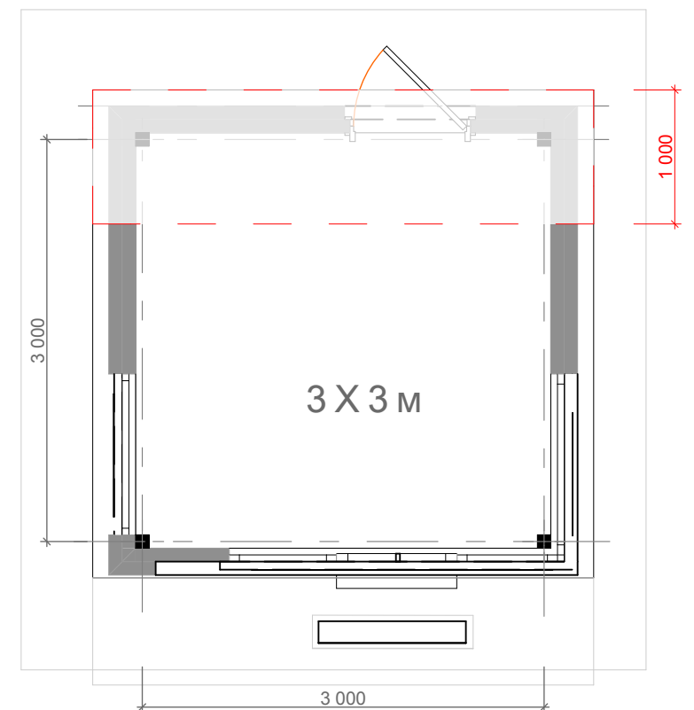
План
