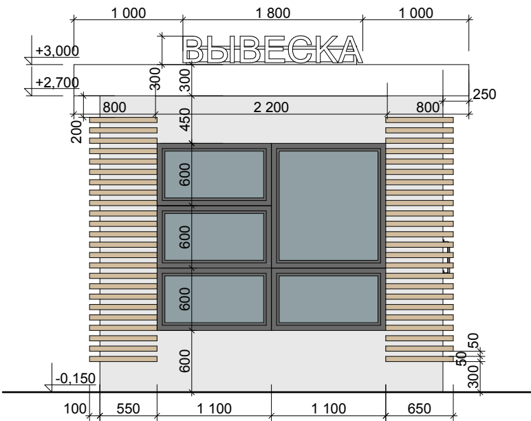
Главный фасад
