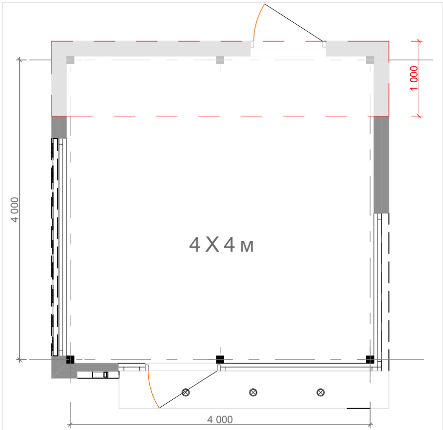
План
