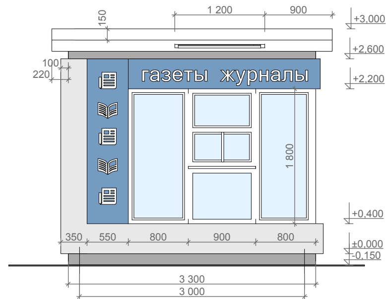
Главный фасад
