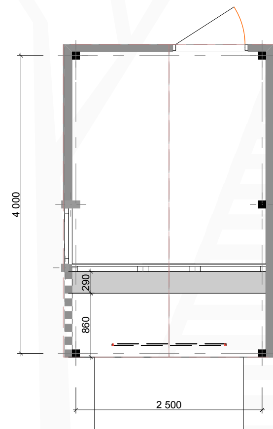
План
