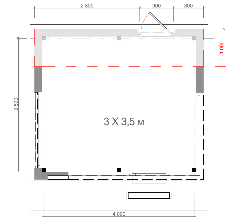
План
