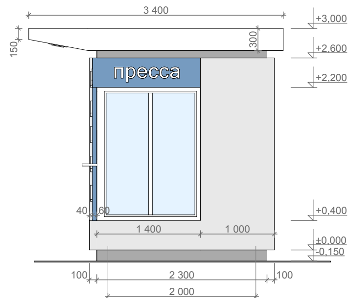
Боковой фасад
