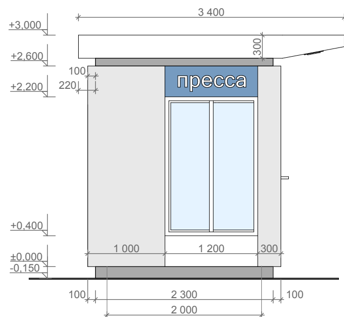
Боковой фасад
