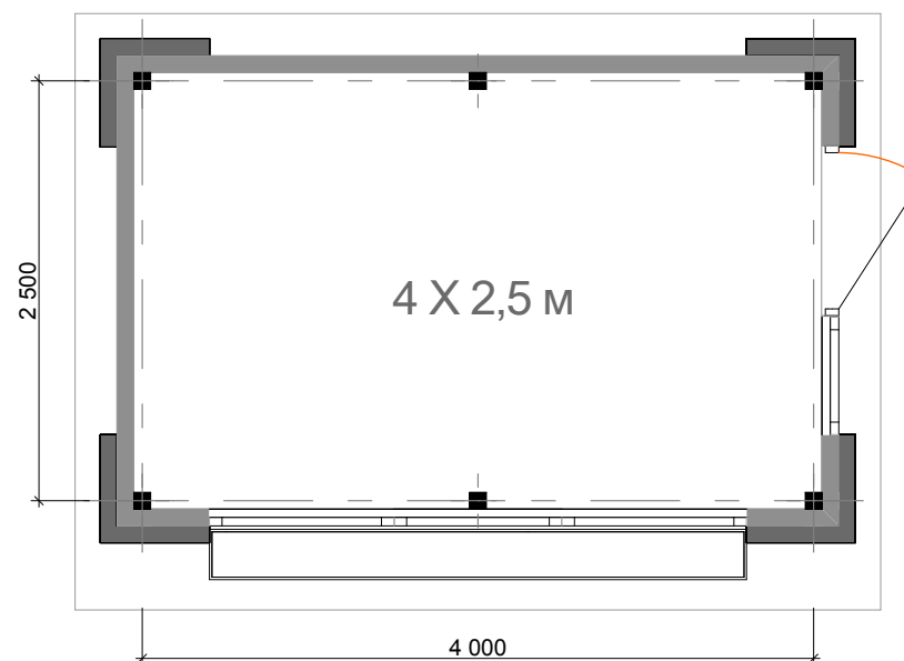
План
