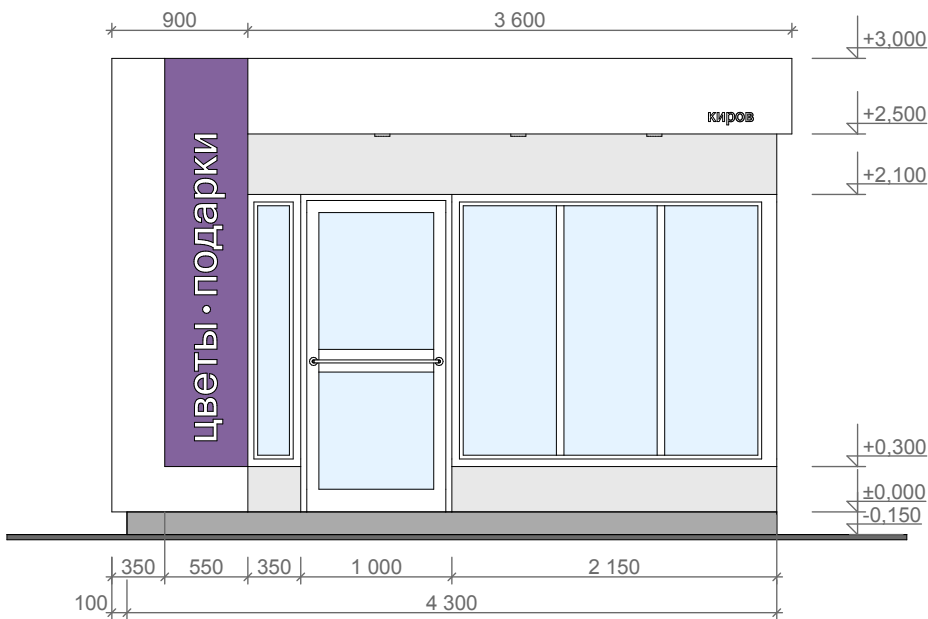
Главный фасад
