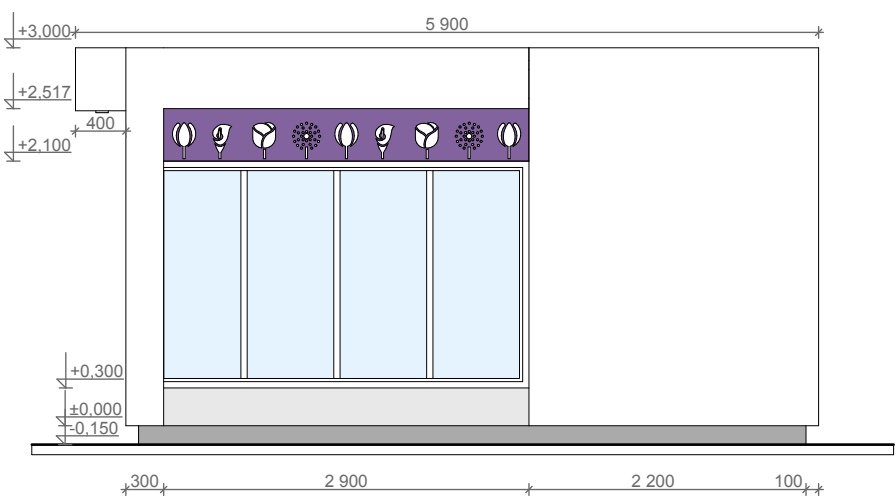
Боковой фасад
