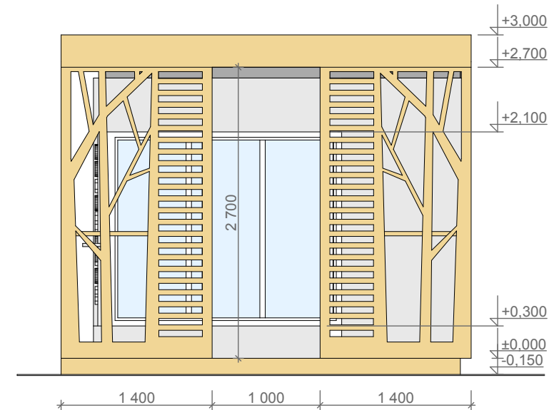
Боковой фасад
