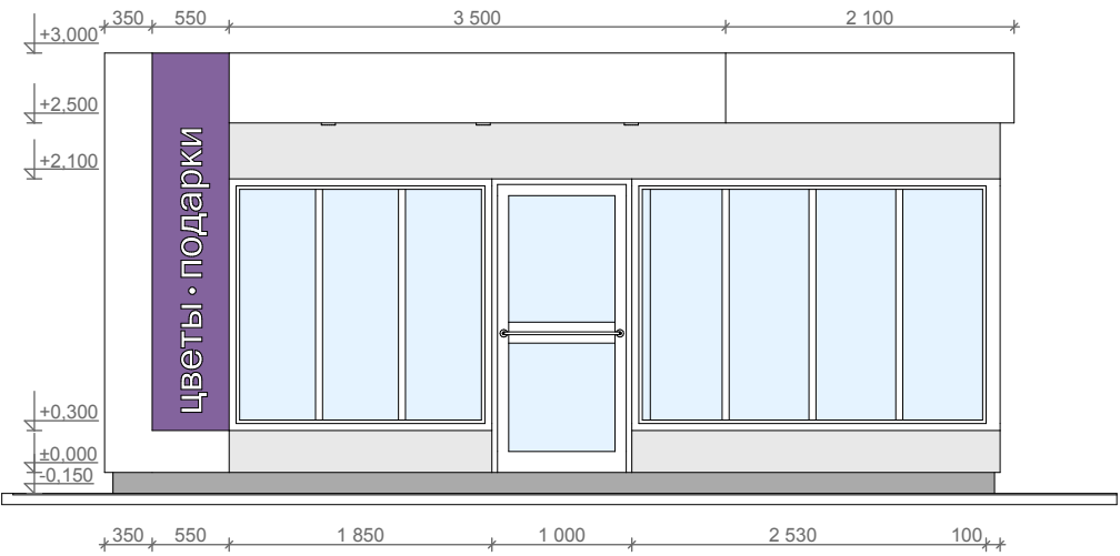
Главный фасад
