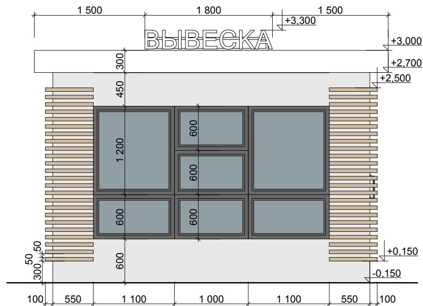
Главный фасад
