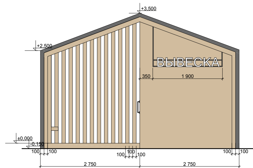
Главный фасад
