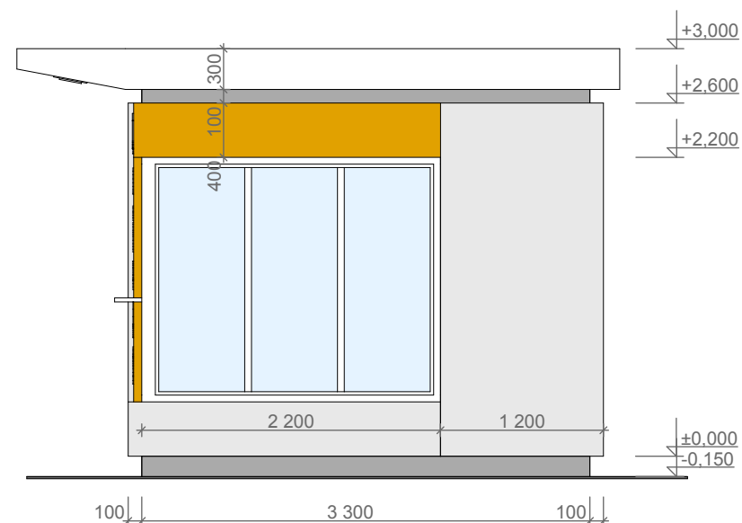
Боковой фасад
