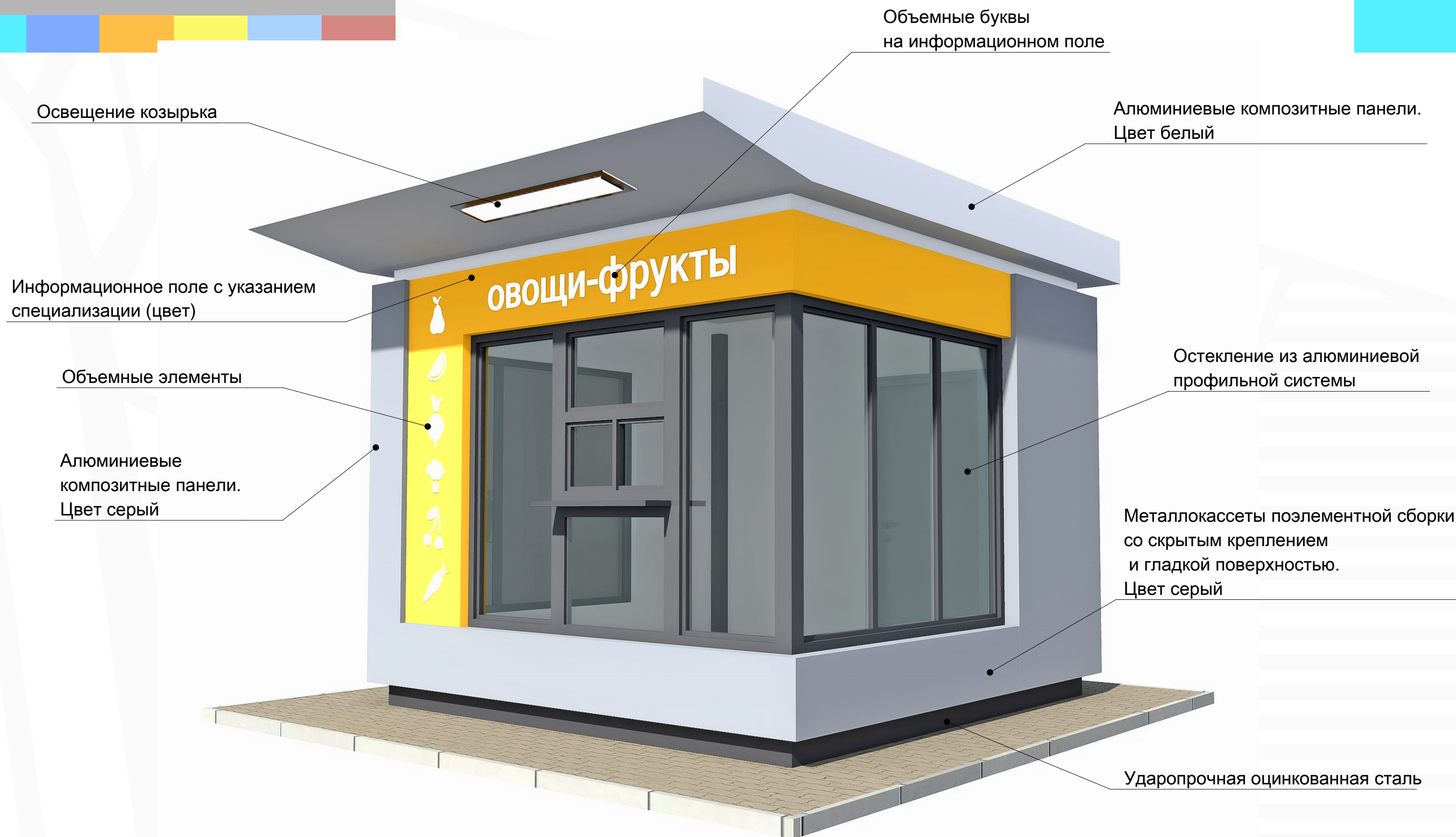
Внешний вид. Вариант с облицовкой композитными панелями для киоска «Овощи-фрукты». Размер в плане 3 x 3 м
