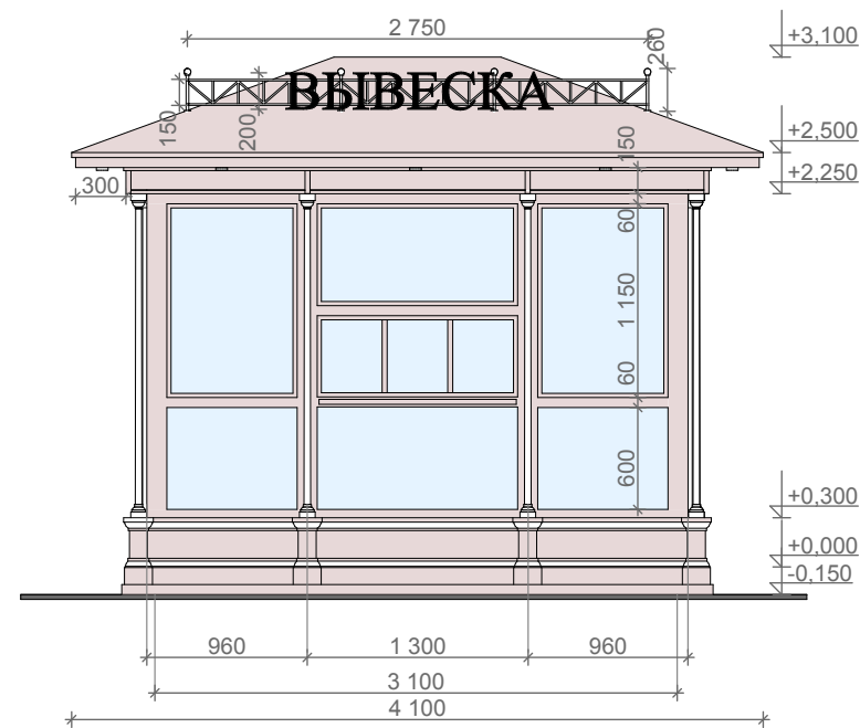
Главный фасад
