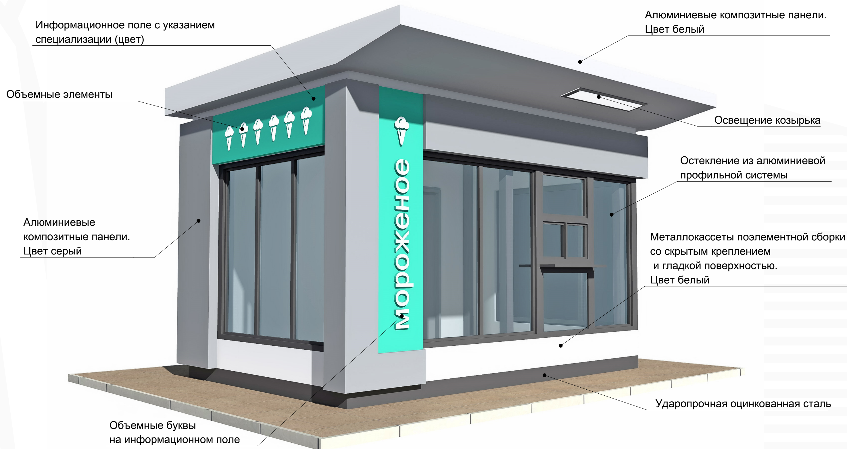
Внешний вид. Вариант с облицовкой композитными панелями для киоска «Мороженое». Размер в плане 4 x 2,5 м
